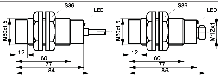
wyjście kablowe
