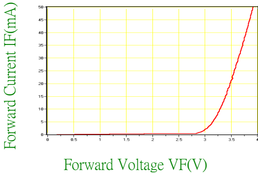
Fig.1 IF-VF(Ta=25°C)
