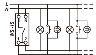
Schemat podłączenia wyłącznika schodowego WS-1S do instalacji 4-przewodowej
