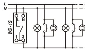
Schemat podłączenia wyłącznika schodowego WS-1S do instalacji 3-przewodowej
