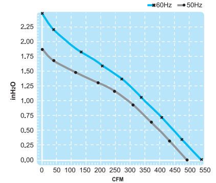
(Centrifugal Fan)
