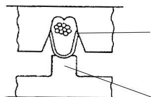
Die geschragten Außenflanken dienen der besseren Führung der Crimphülse in der Obermatritze als auch dem besseren Einrollen der Crimphülsenflanken Better guidance of the crimp barrel in the crimp indenter by the chamfered outer flanks
