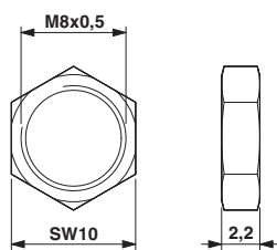
Rysunek wymiarowy
