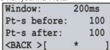
Rysunek 7.5.2. Ekran ustawienia czasu zdarzeniowego zapisu danych
