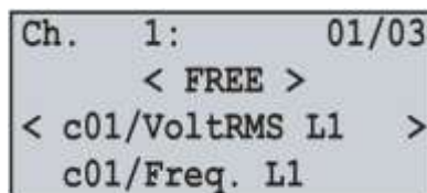
Rysunek 7.4.5. Ekran listy wartości mierzonych
