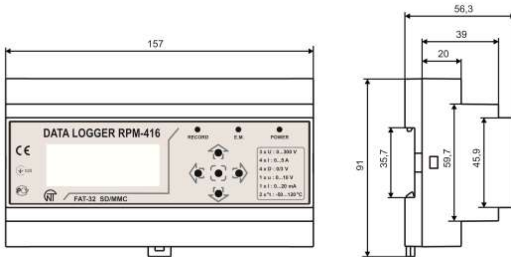
Rysunek 3.1. Wygląd zewnętrzny i wymiary gabarytowe rejestratora
