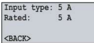
Rysunek 7.2.3. Ekran ustawienia nominalu przekładnika prądowego
