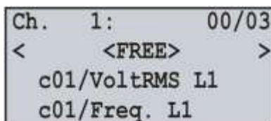
Rysunek 7.5.4. Ekran listy wartości mierzonych
