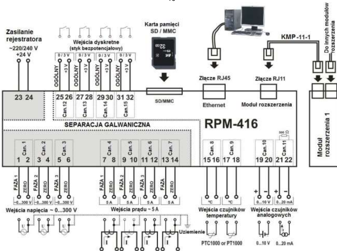
Rysunek 5.1 Schemat podłączenia RPM-416
