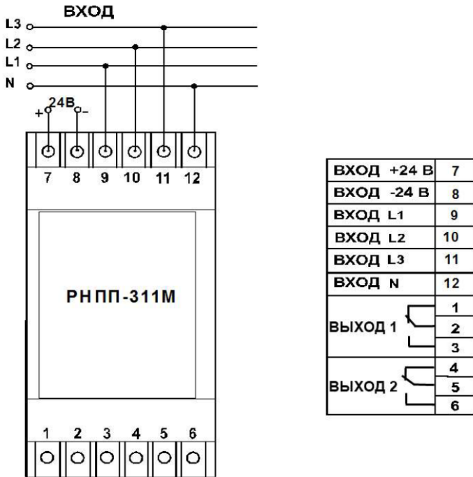
Рисунок 2 - Схема подключения реле РНПП-311М
