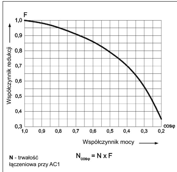
Współczynnik redukcji łączeniowej dla indukcyjnych obciążeń prądu przemiennego
