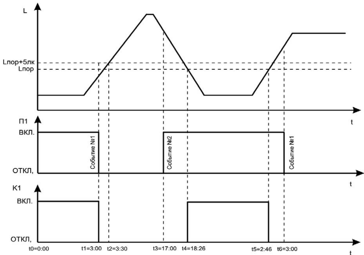
Рисунок 2.10 - Пример совместной работы реле времени и фотореле
