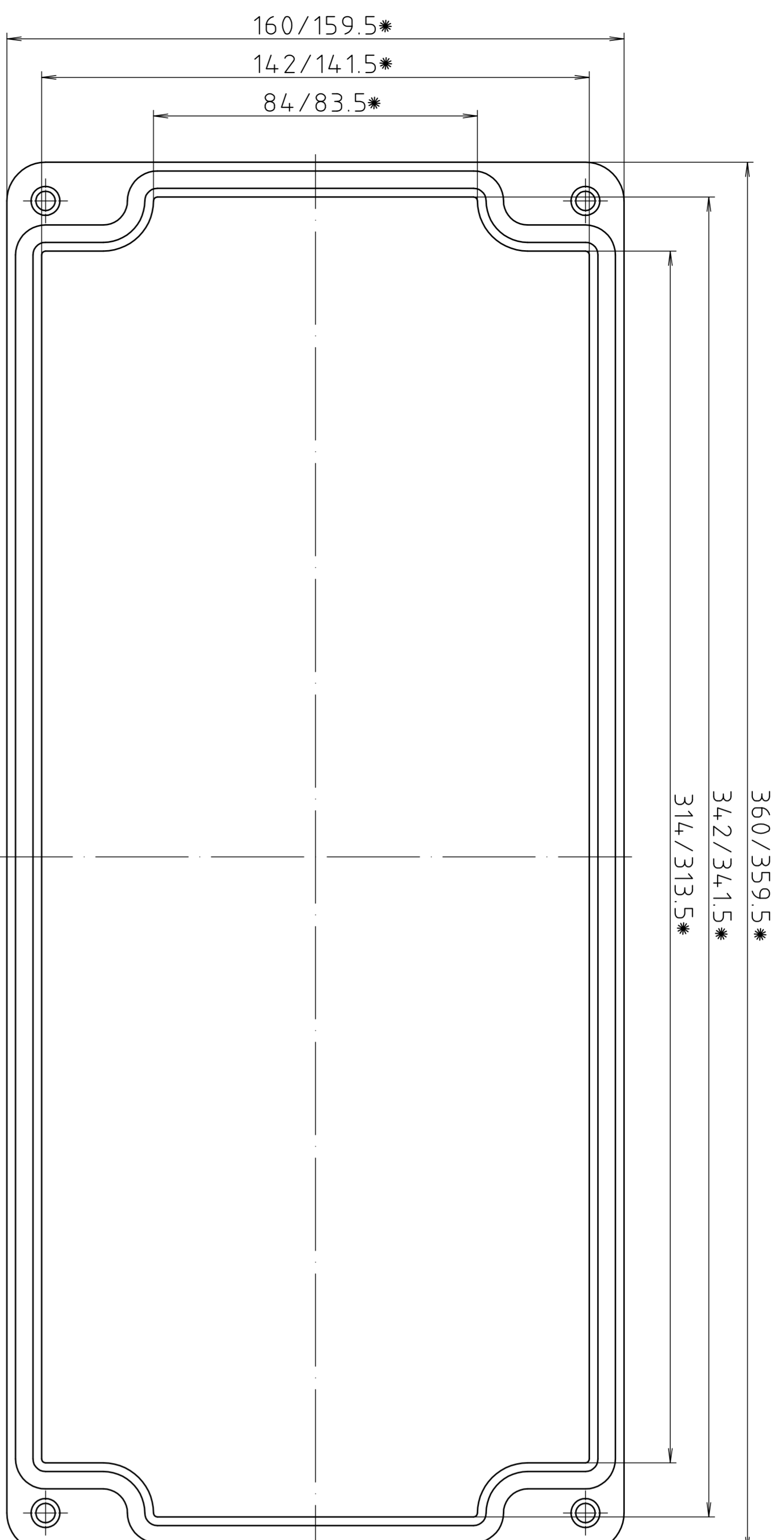
Deckel/ lid
