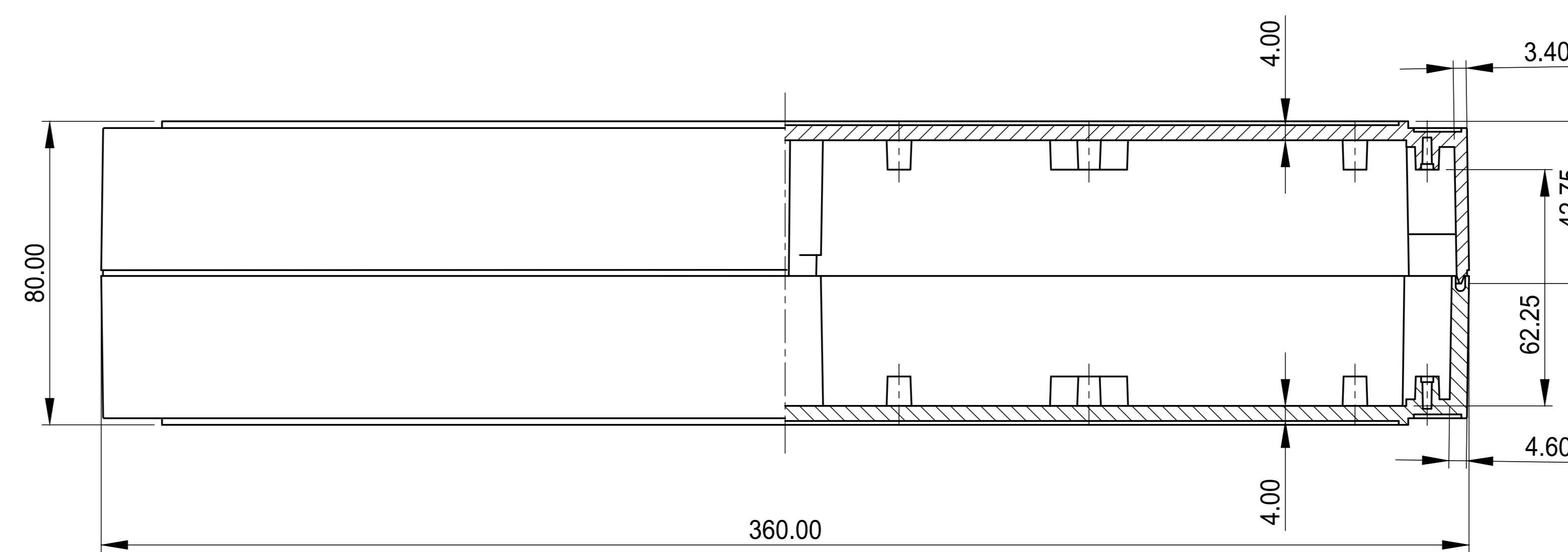
Schnitt A-A section
