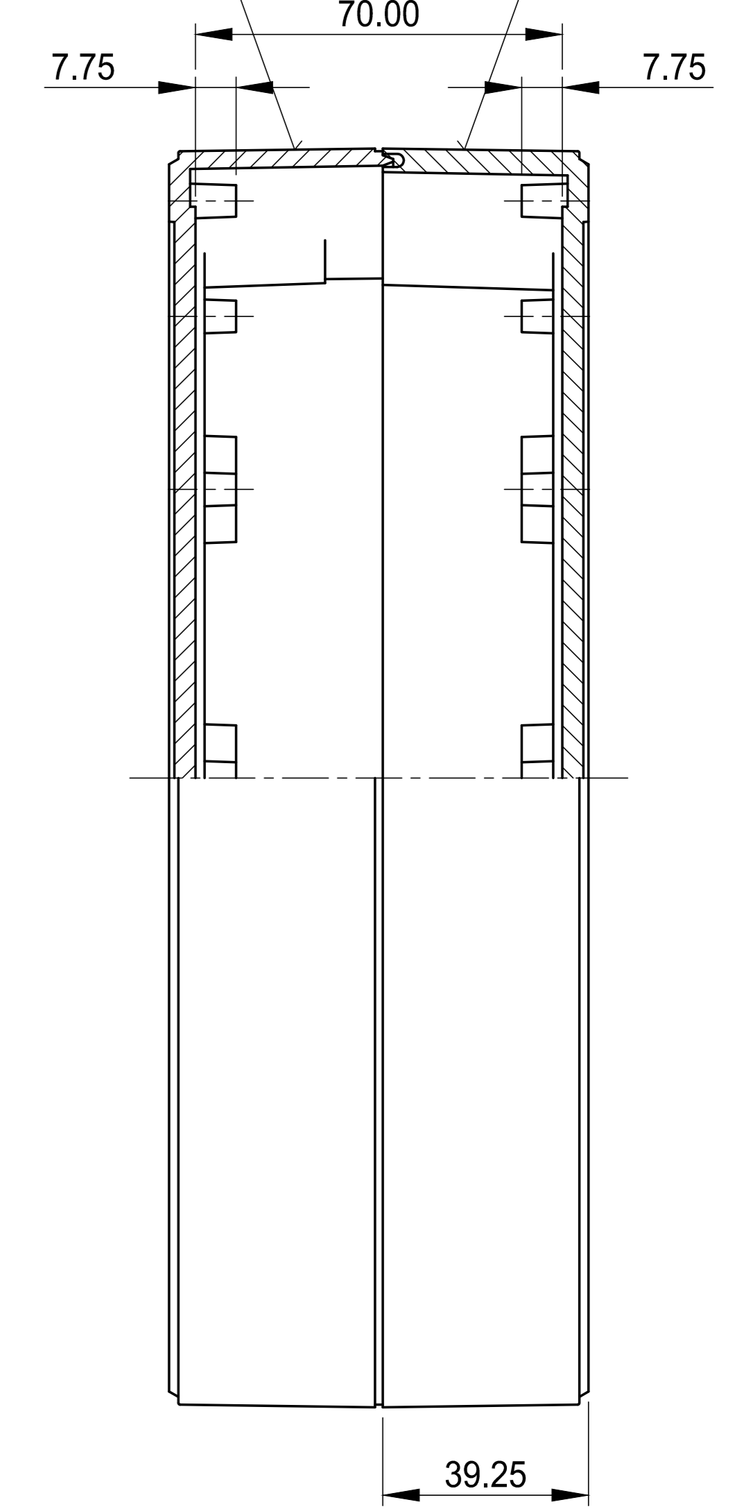
Schnitt B-B section
