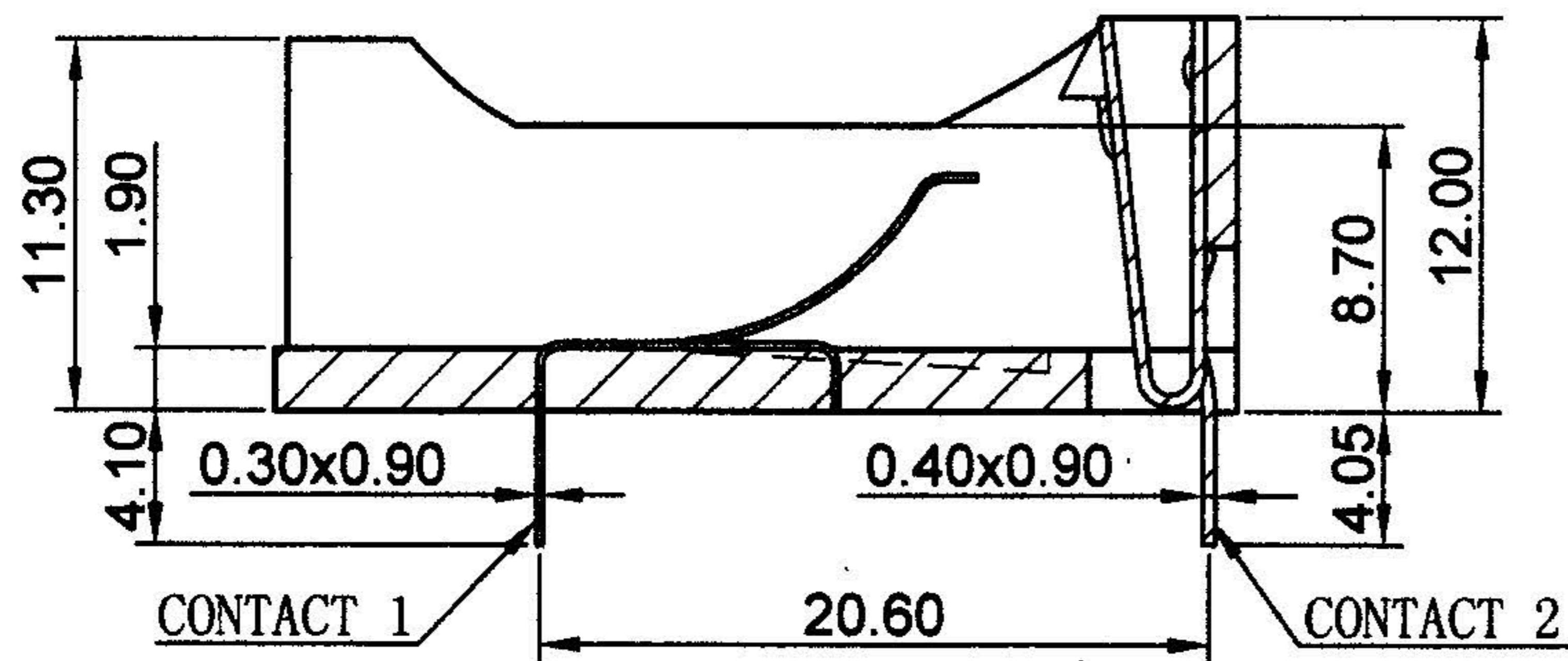
SECTION A-A
