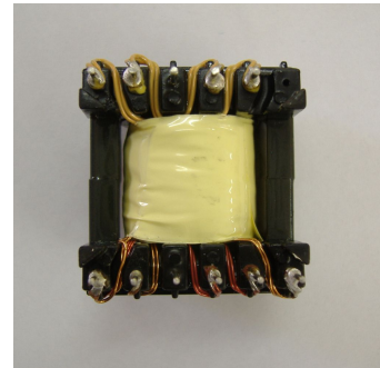
Zdjęcie transformatora
